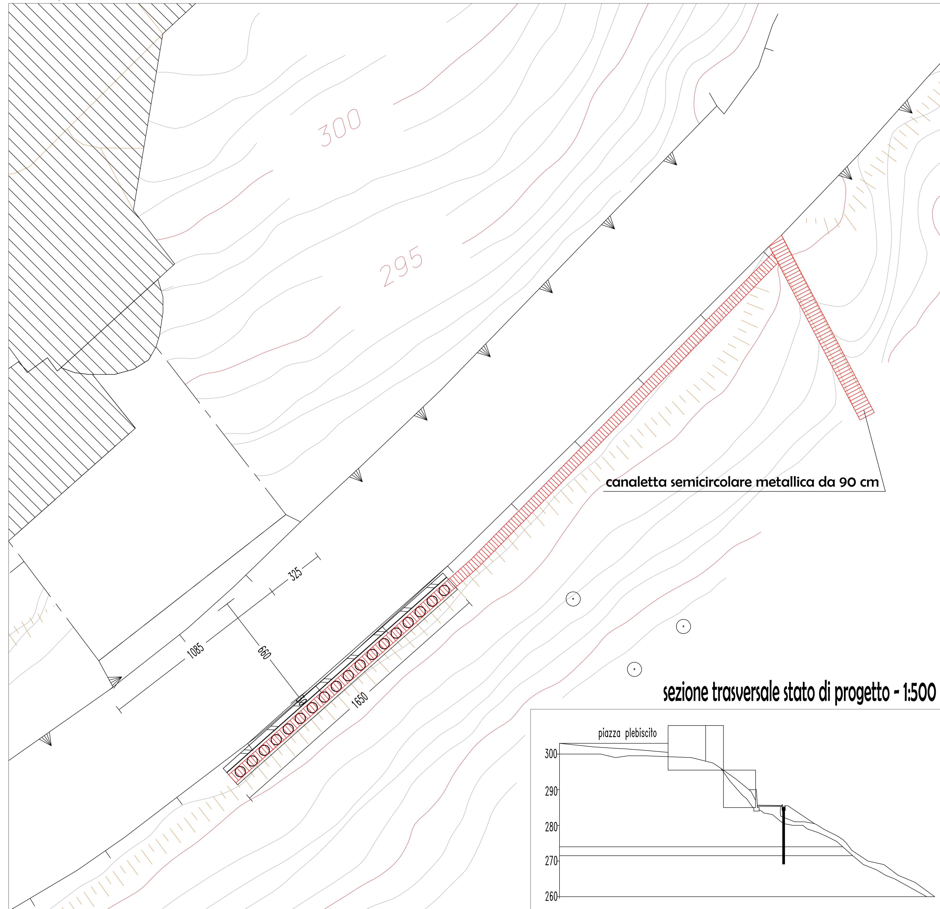
stralcio planimetrico area d'intervento - 1:100
