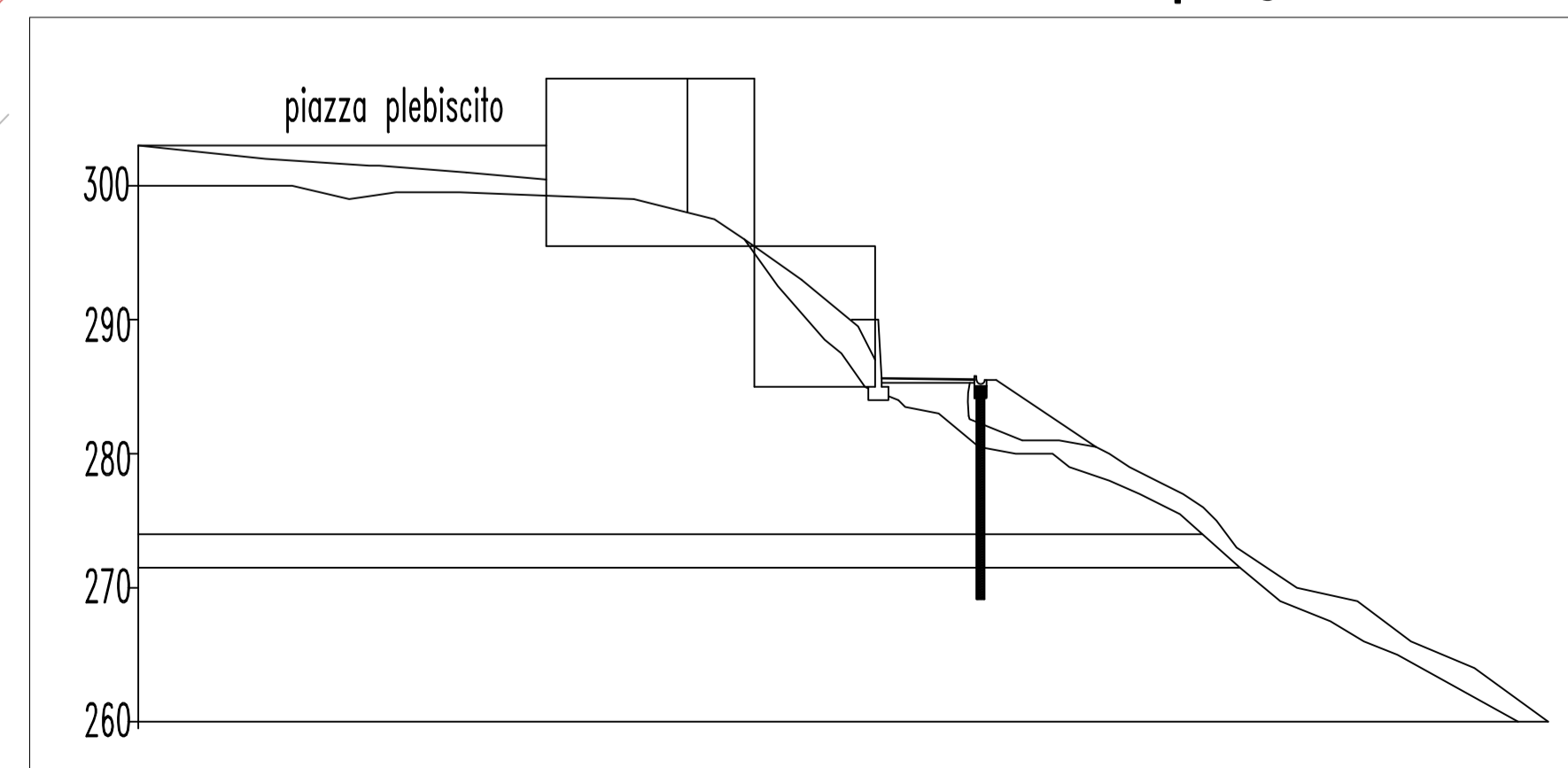
sezione trasversale stato di progetto - 1:500
