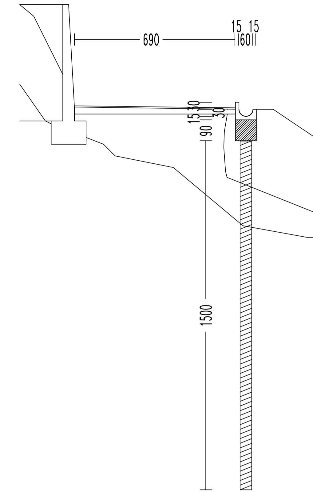
stralcio sezione trasversale - 1:100
